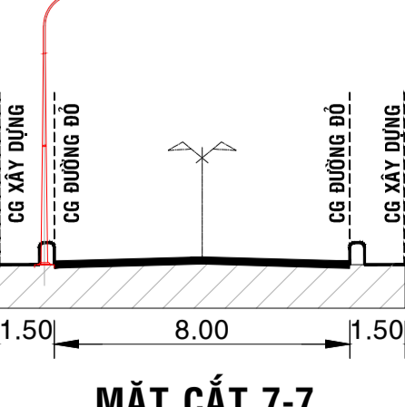
MẶT CẮT 7-7
