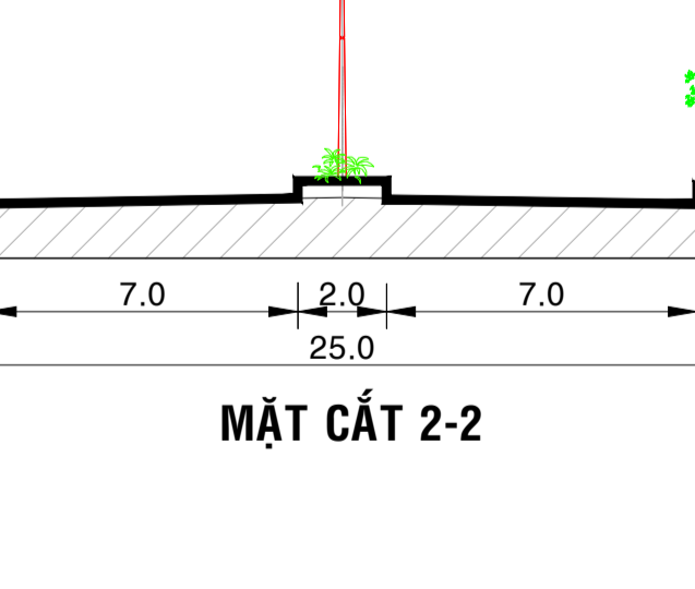
MẶT CẮT 2-2
