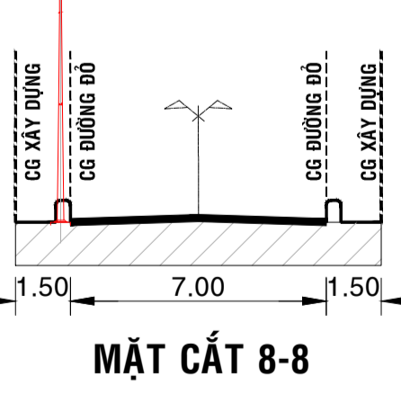
MẶT CẮT 8-8
