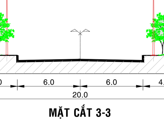
MẶT CẮT 3-3
