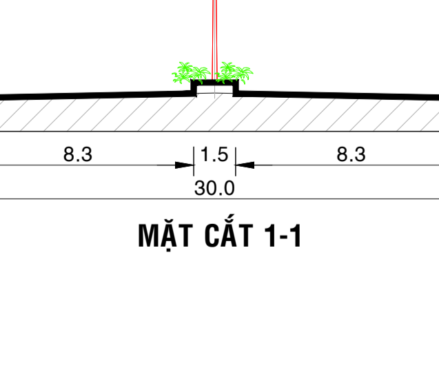
MẶT CẮT 1-1
