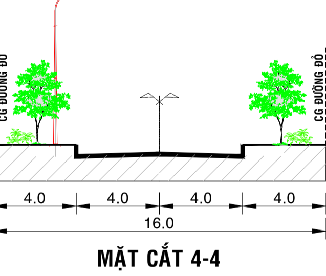
MẶT CẮT 4-4
