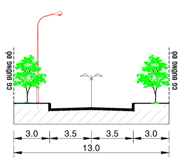
MẶT CẮT 5-5
