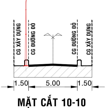
MẶT CẮT 10-10
