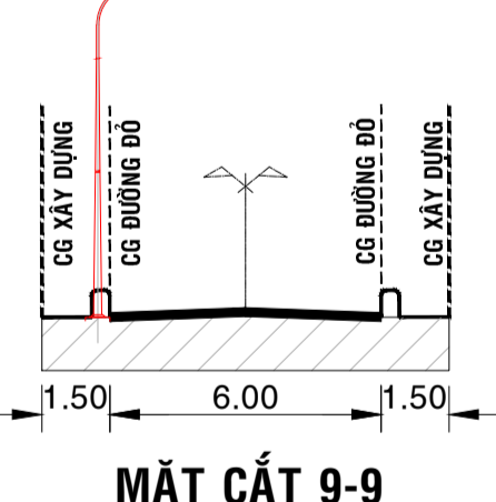
MẶT CẮT 9-9
